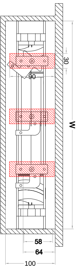
ELEVATION VIEW 正視圖
