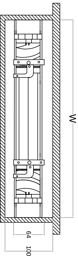
PLAN VIEW 俯視圖
