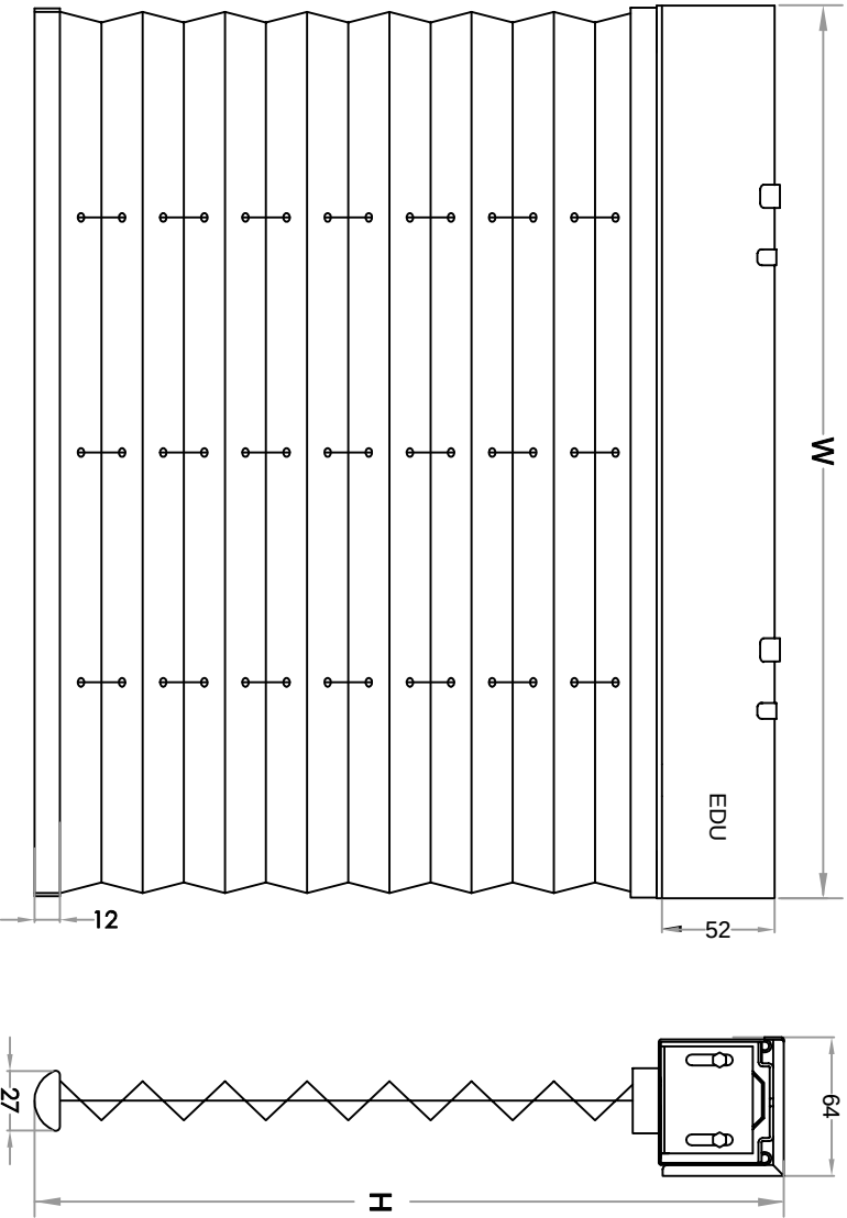
ELEVATION VIEW 正視圖
